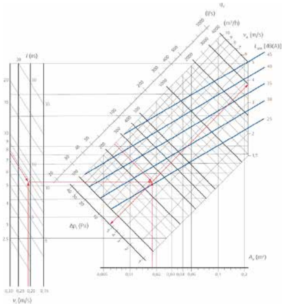
Diagramm 1: Ein Auslegungsdiagramm für die Luftzufuhr für ein zweireihiges Diffusionsgitter bei \Delta t_0 = 0 \text{ °C} und einer horizontalen Luftstromrichtung mit einem Abstand von der Decke von H = 0,2 \text{ m} .
